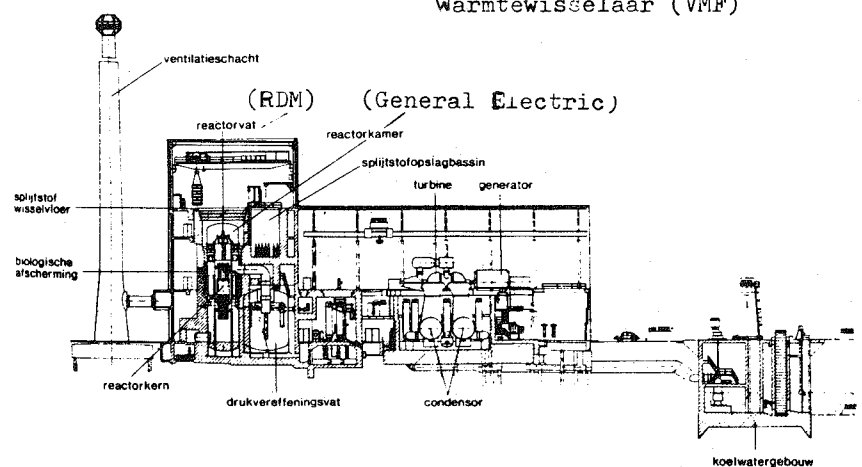
Figuur 2 Dwarsdoorsnede GKN-centrale
